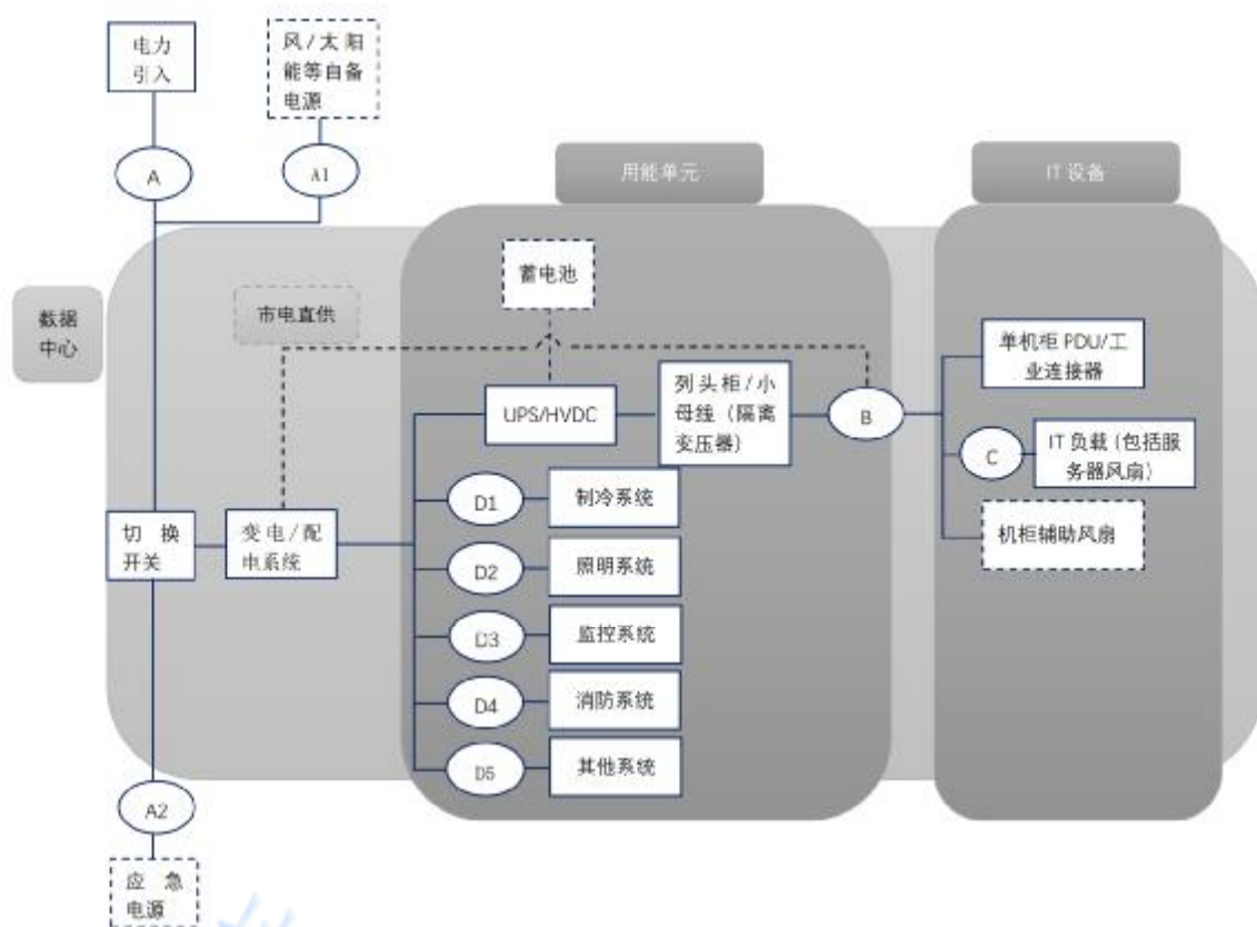
图1 数据中心电能消耗测量点示意图
