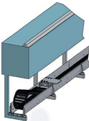
定制的 3D 草图
