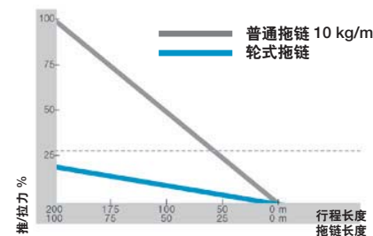
易格斯轮式拖链 5050R 系列用于印度钢厂内，在充满腐蚀性气体的工况中运行着： S = 22 \text{ m} ， a = 1 \text{ m/s}^2
